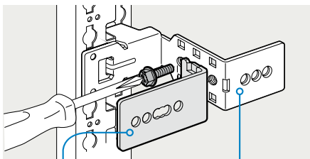
Coté pour montage Vertical
