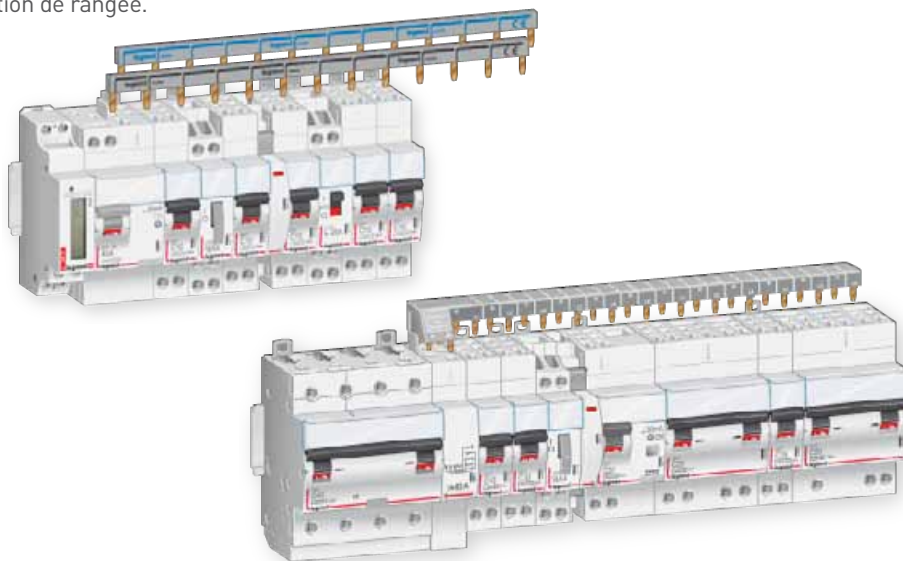
Exemples de raccordements monophasé et triphasé
