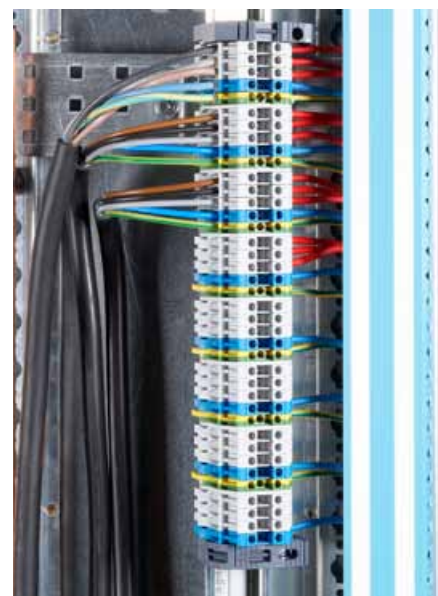
Exemple de réalisation d'un bornier vertical à l'aide du support universel pour gaines à câbles interne réf. 0 201 96
