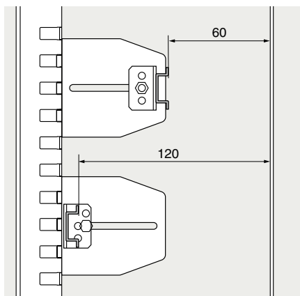
Distances minimum et maximum entre rail réf. 0 206 02/52 et plastron
