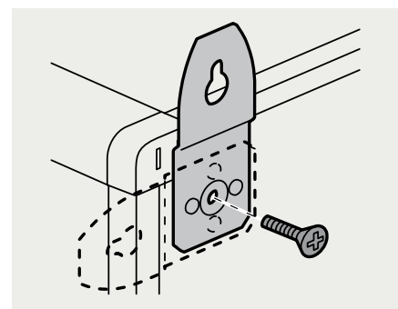
Visser ensuite la patte dans la position souhaitée
