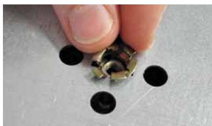
Enlever le cache plastique à l'arrière de l'armoire et mettre en place du clip-écrou
